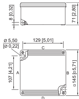
8118/.3. Enclosure SZ 3
